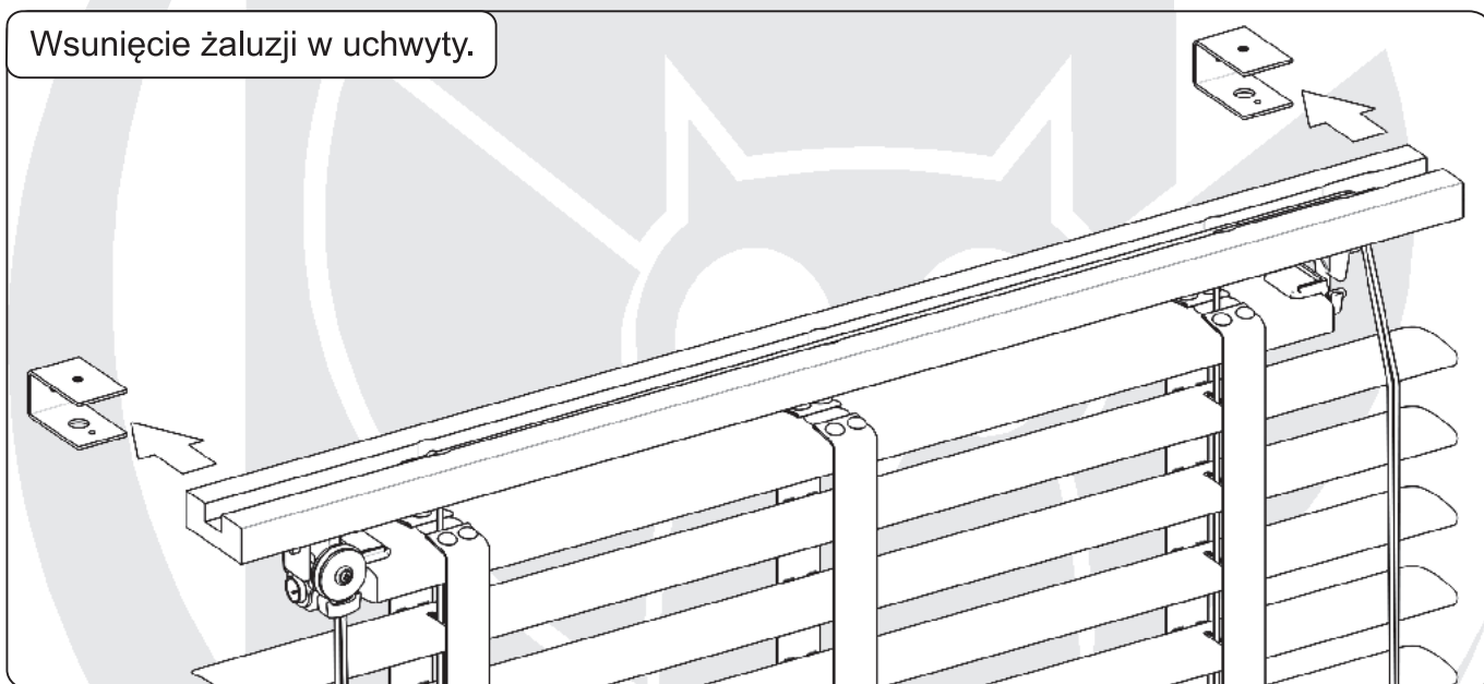
Przykręcenie żaluzji.
