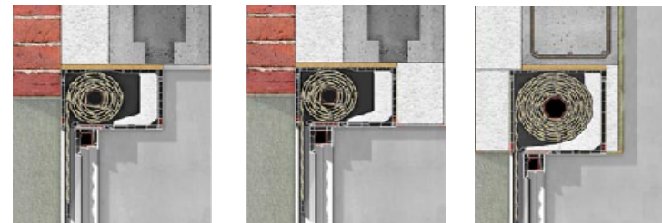
Typ montażu: A - bez zabudowy B - z zabudową od wew. C - z zabudową całkowitą
