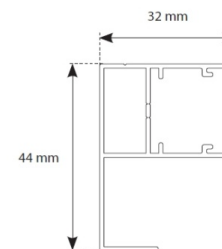
Rys. 3 Prowadnica z odsadzeniem
