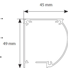
Rys. 1 Przekrój skrzynki
