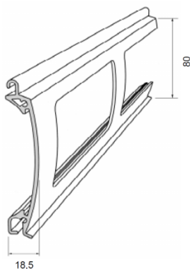
profil PEK80
